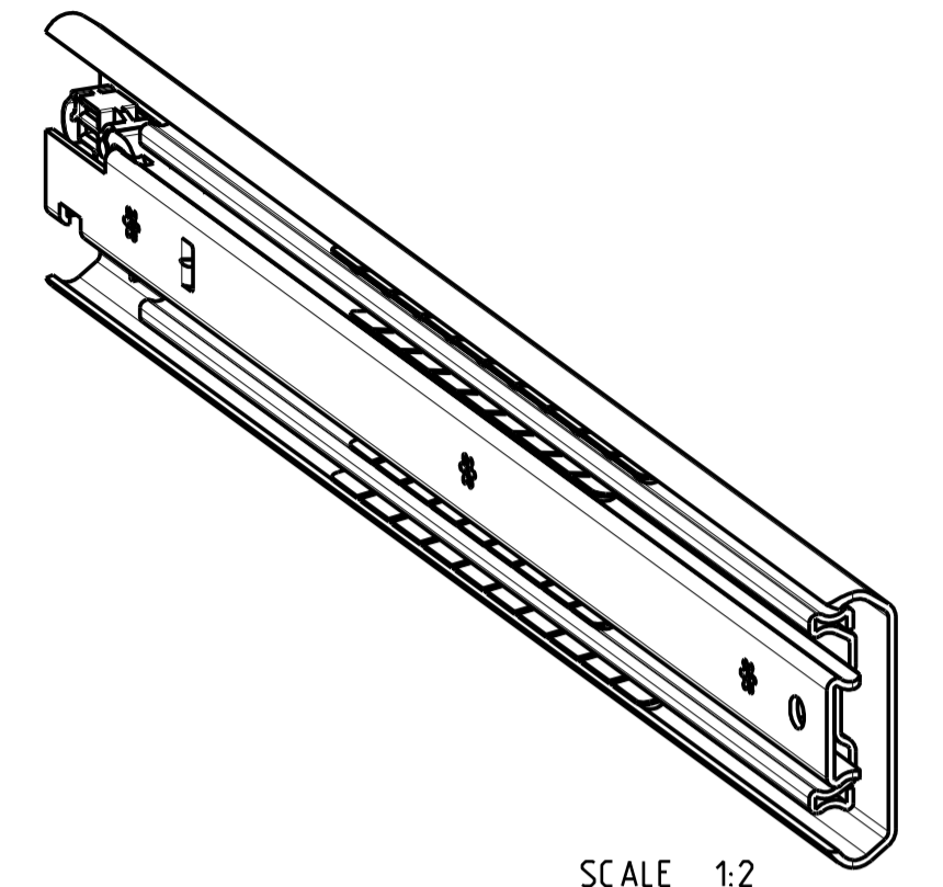
SCALE 1:2
