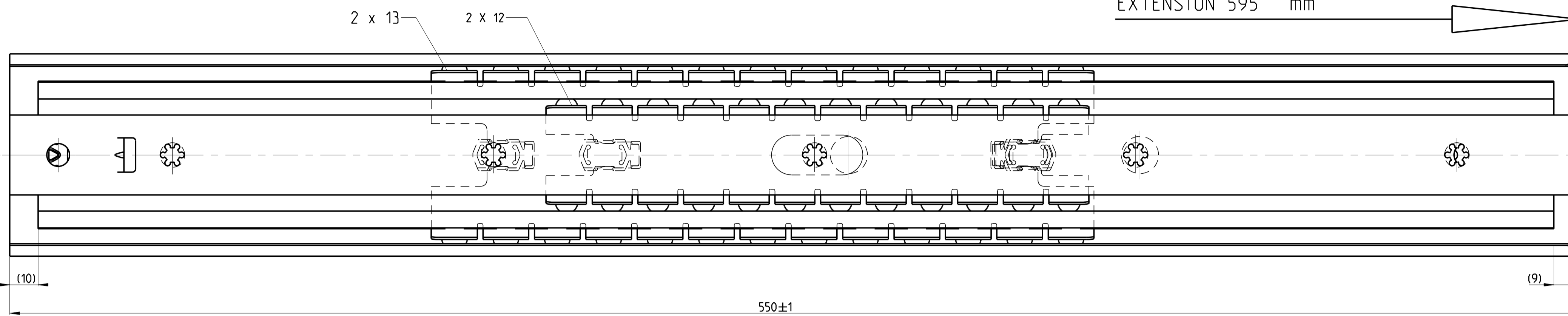
SECTION A-A
